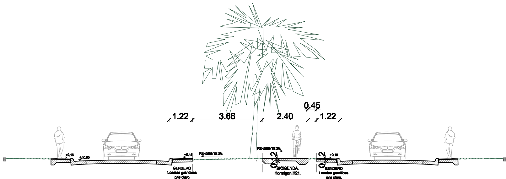
CORTE A
