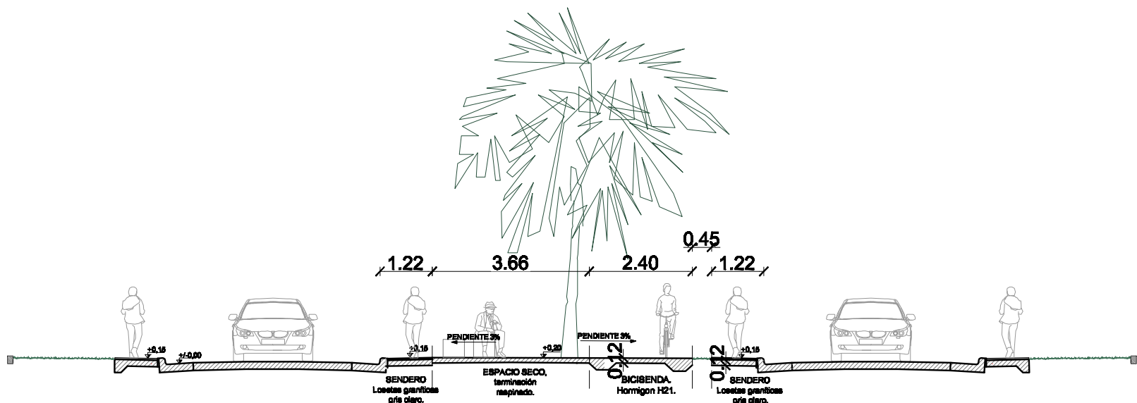
CORTE B
